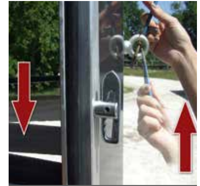
Barre de poitrail de sécurité avec boucle de sécurité extérieure.
